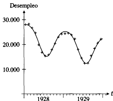
FIGURA 4.10 Una curva lisa que aproxima los puntos de la Figura 4.9
