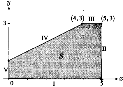
FIGURA 17.8 Dominio del Ejemplo 17.6.
