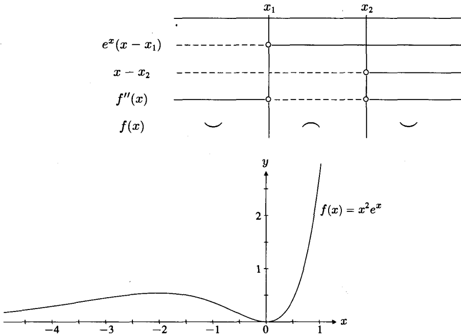
FIGURA 9.22 f(x) = x^2 e^x
