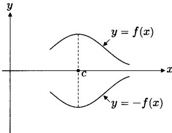
FIGURA 9.1: El punto c es un máximo de f(x) y uno de mínimo de -f(x) .
