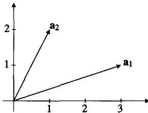
FIGURA 14.2 Los vectores \mathbf{a}_1 y \mathbf{a}_2 son linealmente independientes.
