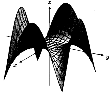
FIGURA 15.13 z = x^4 - 3x^2y^2 + y^4 .
