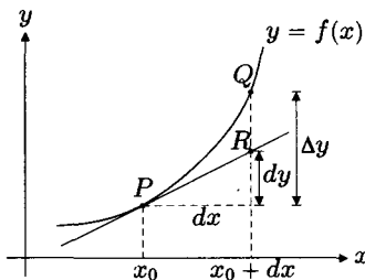
FIGURA 5.3 Representación geométrica de la diferencial.
