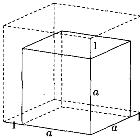
FIGURA 2.3 Volumen f(a+1) = (a+1)^3 :
