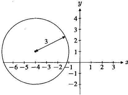
FIGURA 2.18 Circunferencia de centro (-4, 1) y radio 3.
