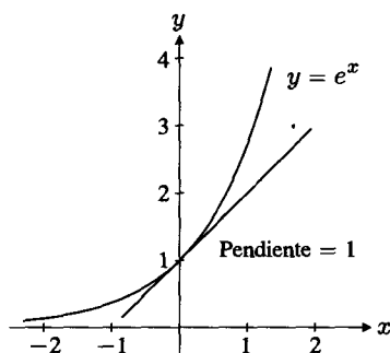
FIGURA 8.3 La función exponencial natural.
