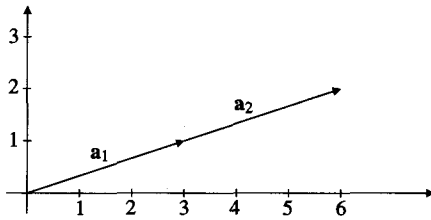
FIGURA 14.1 Los vectores \mathbf{a}_1 y \mathbf{a}_2 son linealmente dependientes.
