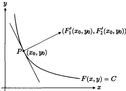
FIGURA 16.3 El gradiente es ortogonal a la tangente en P .
